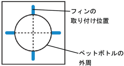
フィン取り付け位置図
